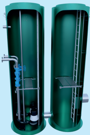
Насосная станция многокорпусная
